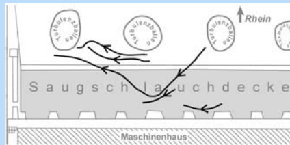
Dokumentiertes Strömungsbild
