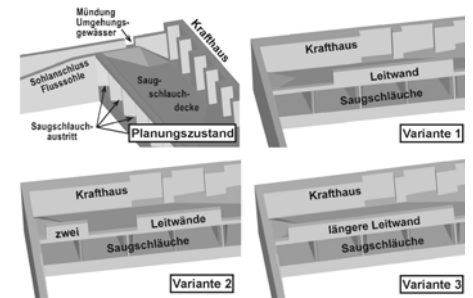
Bauwerksgeometrie mit Mündung des Umgehungsgerinnes sowie bauliche Veränderungen
