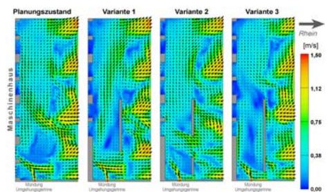
Berechnete Strömungszustände über der Saugschlauchdecke (horizontale Schnitte)
