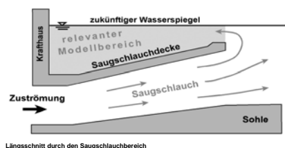
Längsschnitt durch den Saugschlauchbereich
