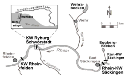
Lageplan der Stauhaltung
