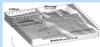
Modellgeometrie des 3D-HN-Modells
