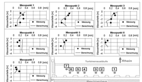
Vergleich von gemessenen und berechneten Strömungsgeschwindigkeiten über der Saugschlauchdecke
