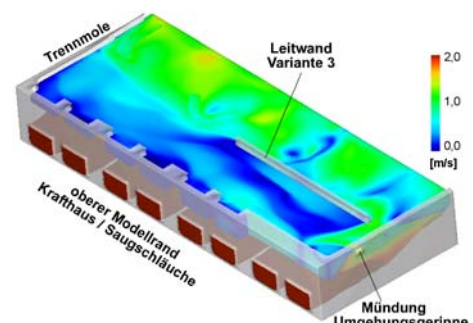
Dreidimensionale Ansicht des berechneten Strömungszustands bei Variante 3
